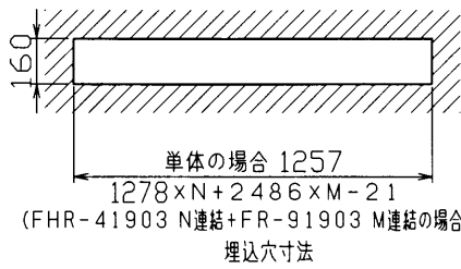
埋込穴寸法
