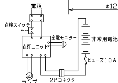
結線図
