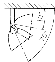
天井取付 下向き10度 照射範囲 下向き70度の間
