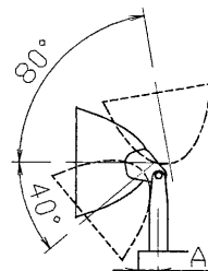
水平取付 上向き80度 照射範囲 下向き40度の間
