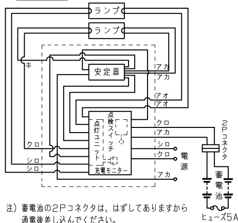
結 線 図
