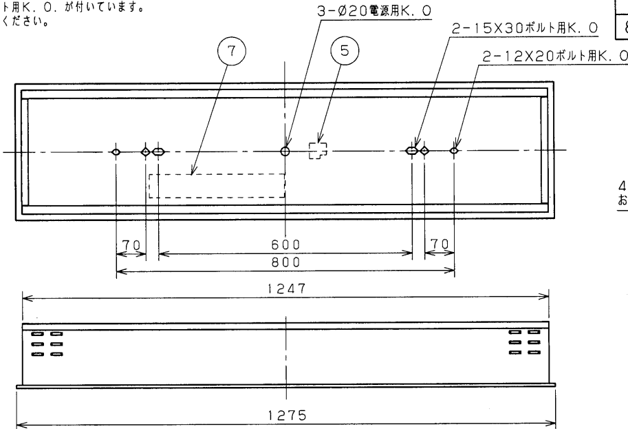
取付けボルトの器具内寸法
