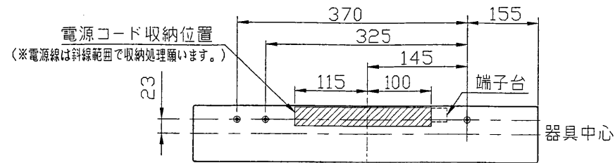
器具中心 取付寸法図
