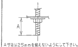
取付ボルトの器具内寸法
