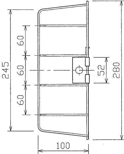
壁直付専用
