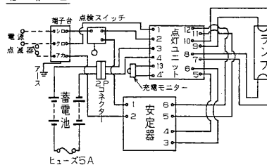
結線図
