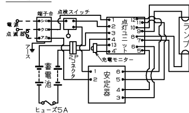
結 線
