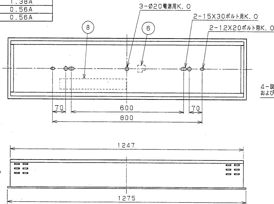
取付ボルトの器具内寸法
