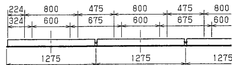
埋込連結使用例
