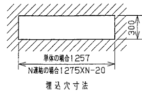
埋込穴寸法
