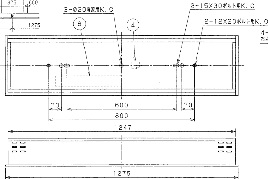
埋込連結使用例
