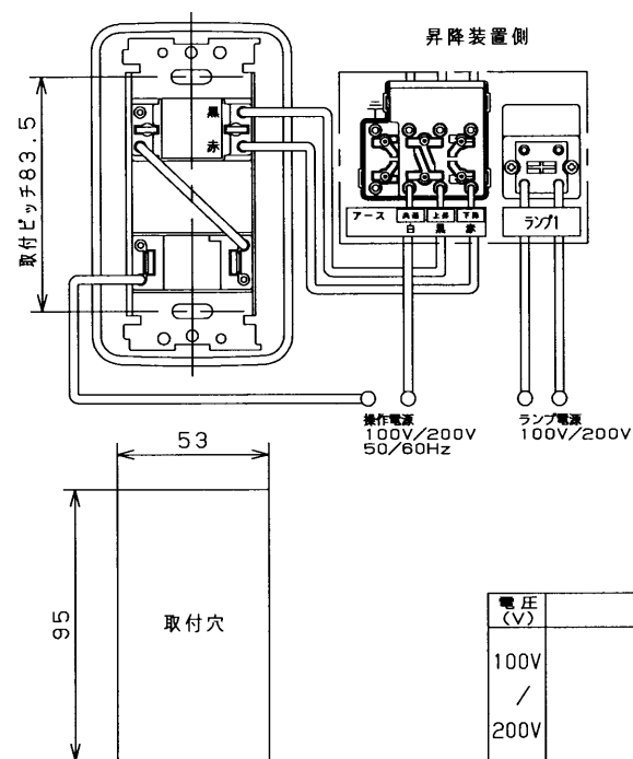
結線図
