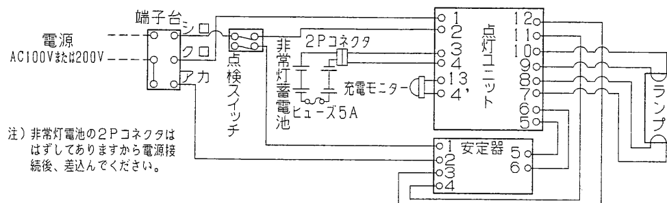
結線図
