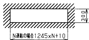
埋込寸法
