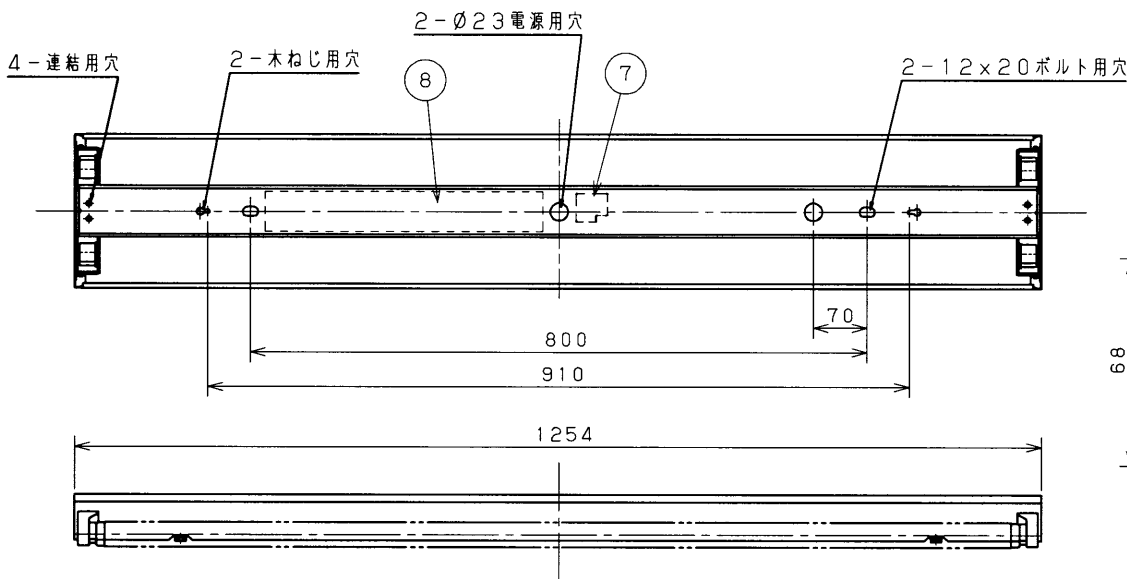
直付連結使用例
