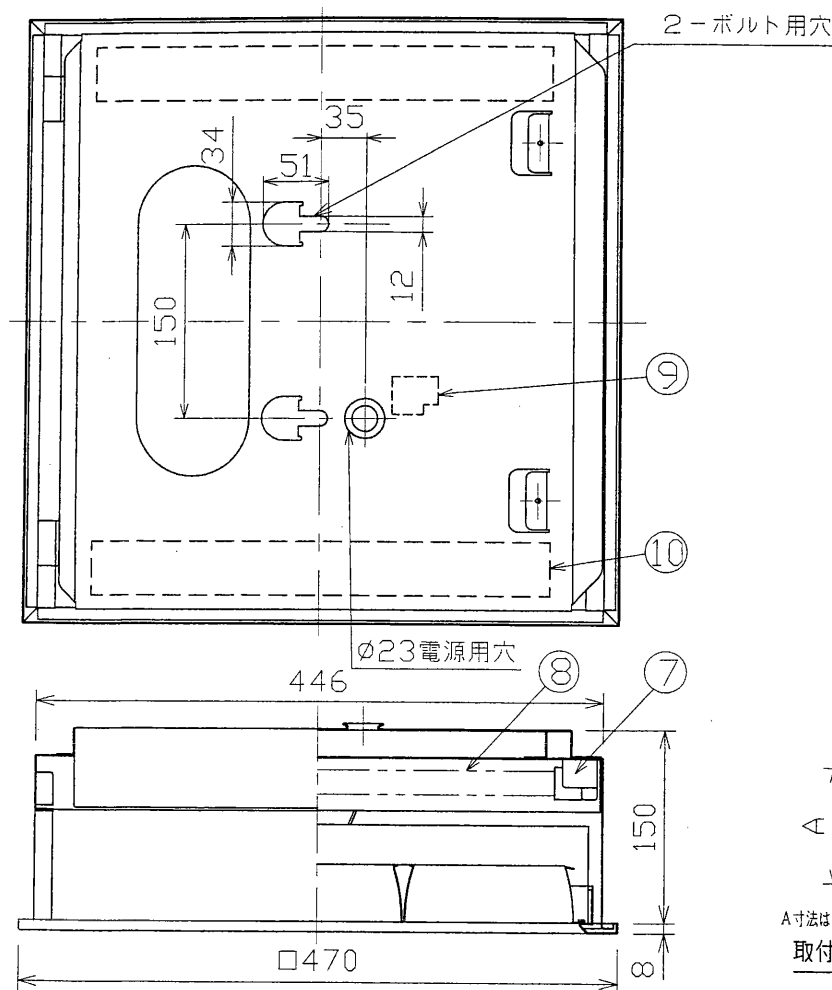
埋込穴寸法
