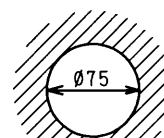
埋込穴寸法 天井取付厚さ: 5~25mm
