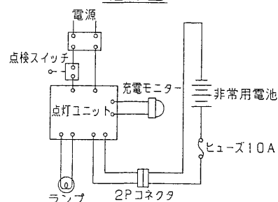
結線図
