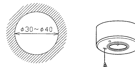
電源穴寸法
