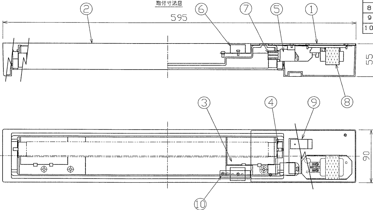
取付寸法図
