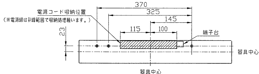
取付寸法図
