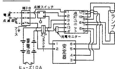
結線図
