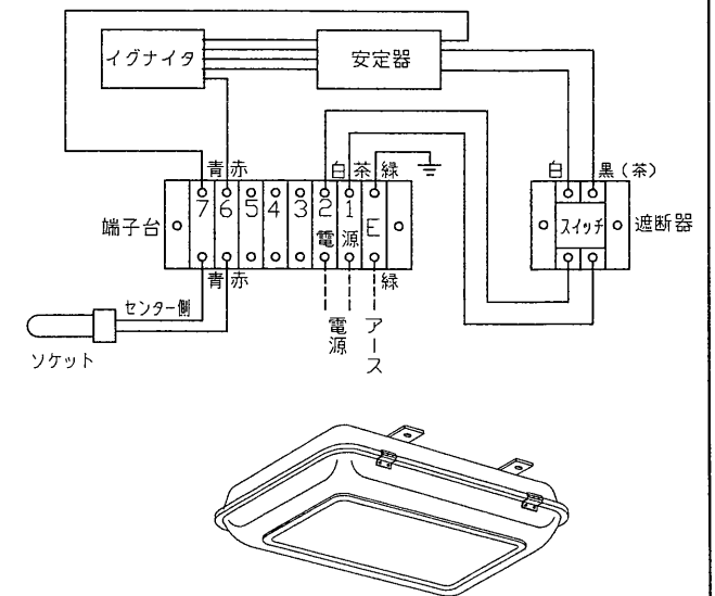
結線図
