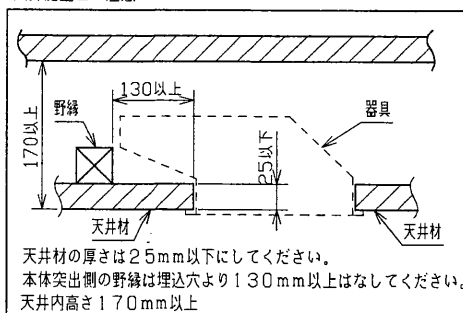
天井施工上の注意
