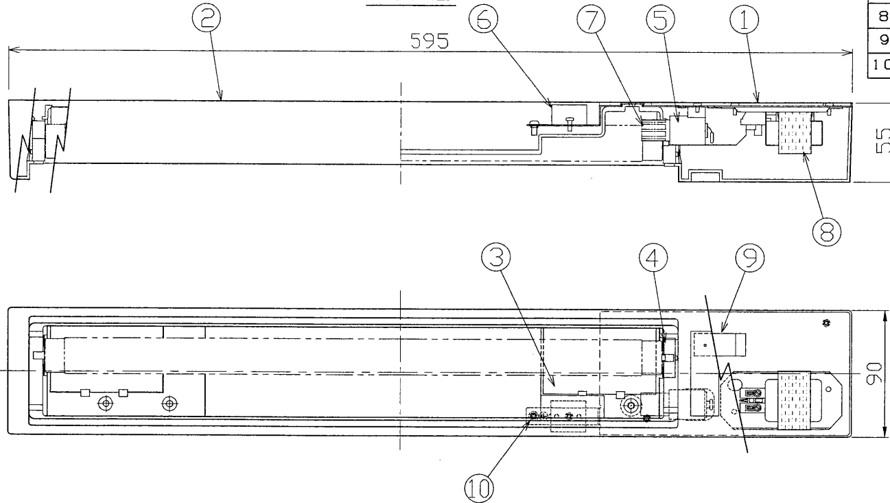
器具中心 取付寸法図
