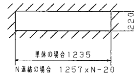
埋込穴寸法
