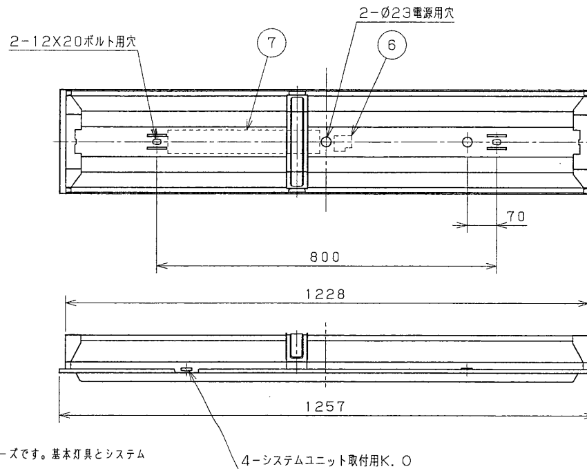
埋込穴寸法
