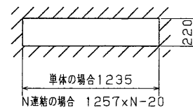
埋込穴寸法
