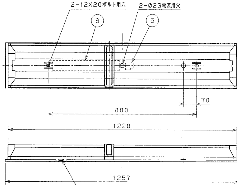
埋込穴寸法
