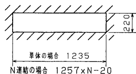
埋込穴寸法
