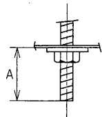
取付ボルトの器具内寸法
