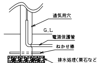
ねかせ棒仕様の施工の場合
