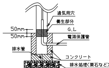
コンクリート施工の場合
