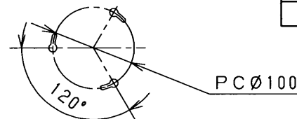
安定器ボックス取付ピッチ
