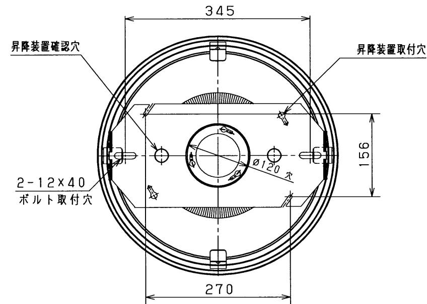
安定器ボックス取付ピッチ
