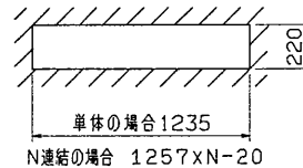
埋込穴寸法
