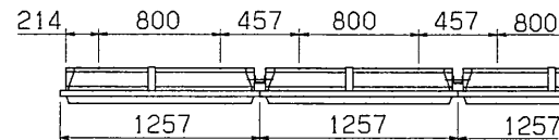
連結使用例
