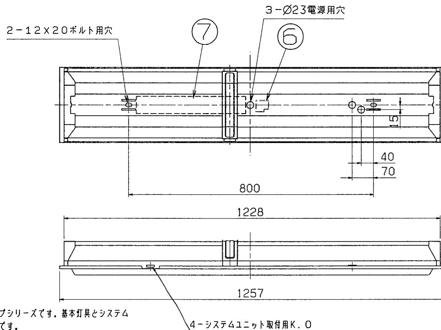
埋込穴寸法
