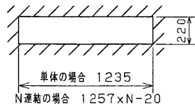
埋込寸法
