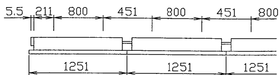
連結使用例
