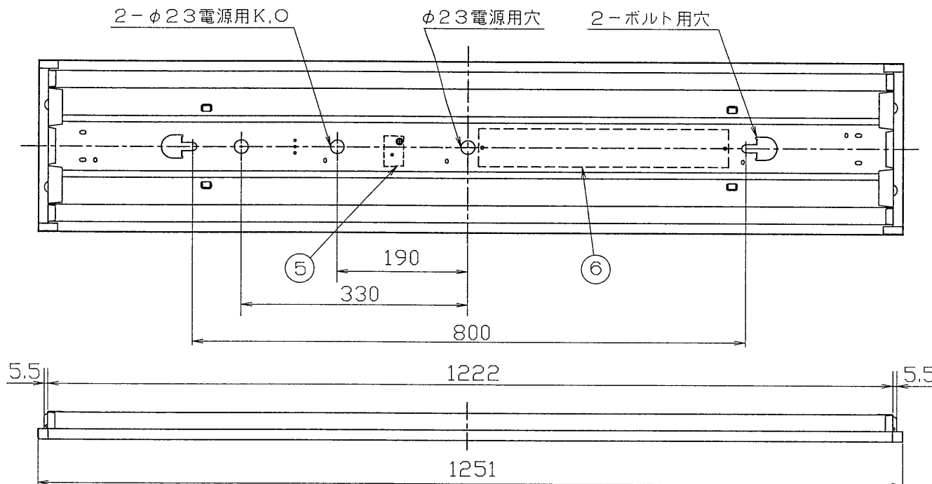
埋込穴寸法
