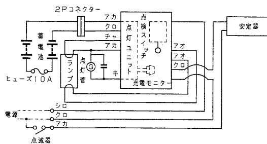
結線図
