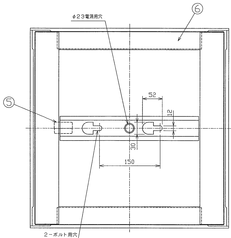
インサートボルト(器具取付ボルト)器具内寸法 注) A寸法は、30mmを超えないようにしてください。
