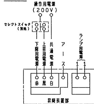
結線図
