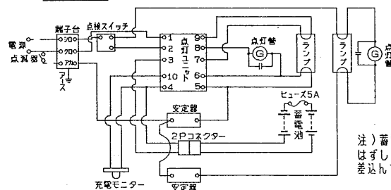
結線図
