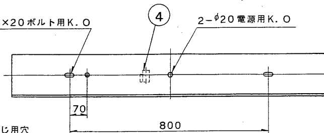
B 矢 視 図
