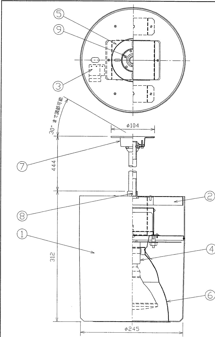
取付寸法図
