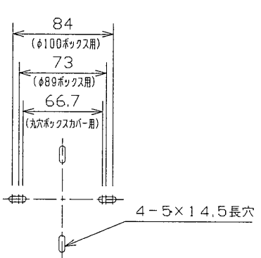
取付寸法図
