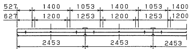
直付連結使用例
