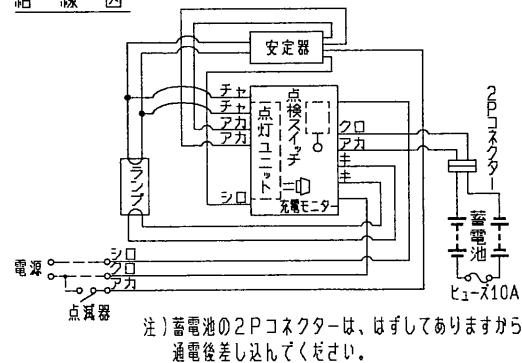
結線図
