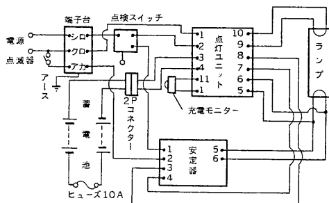
結線図
