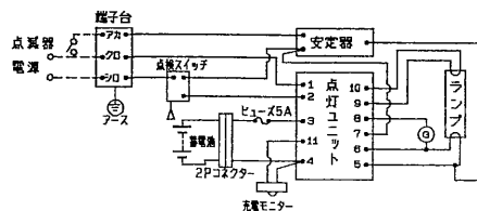
結 線 図
