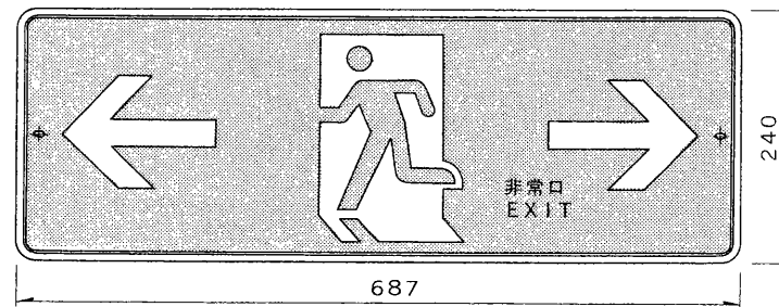
ET-2043
