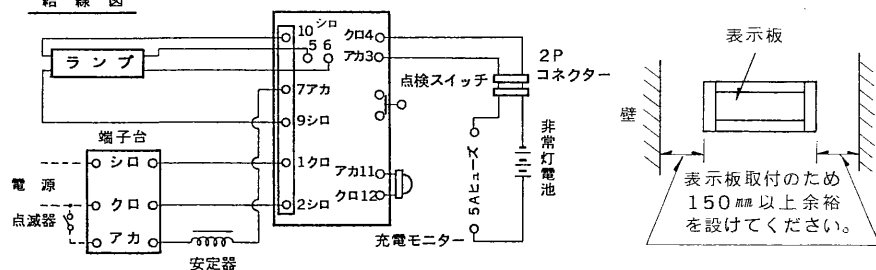
結線図
