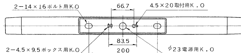
天井直付の場合：取付け寸法図
