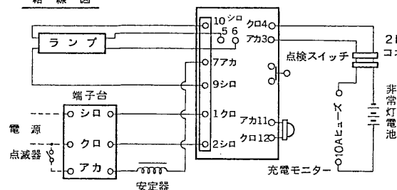
結 線 図
