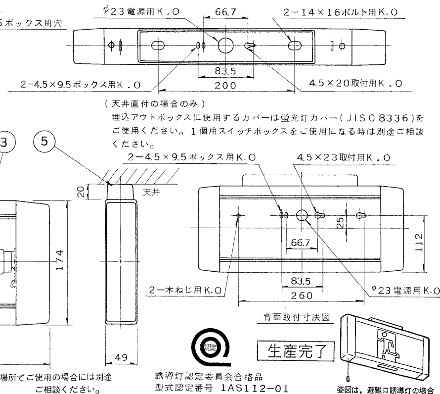
天井直付の場合：取付け寸法図
