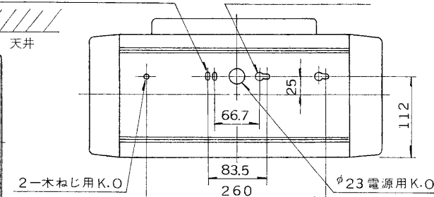
背面取付寸法図
