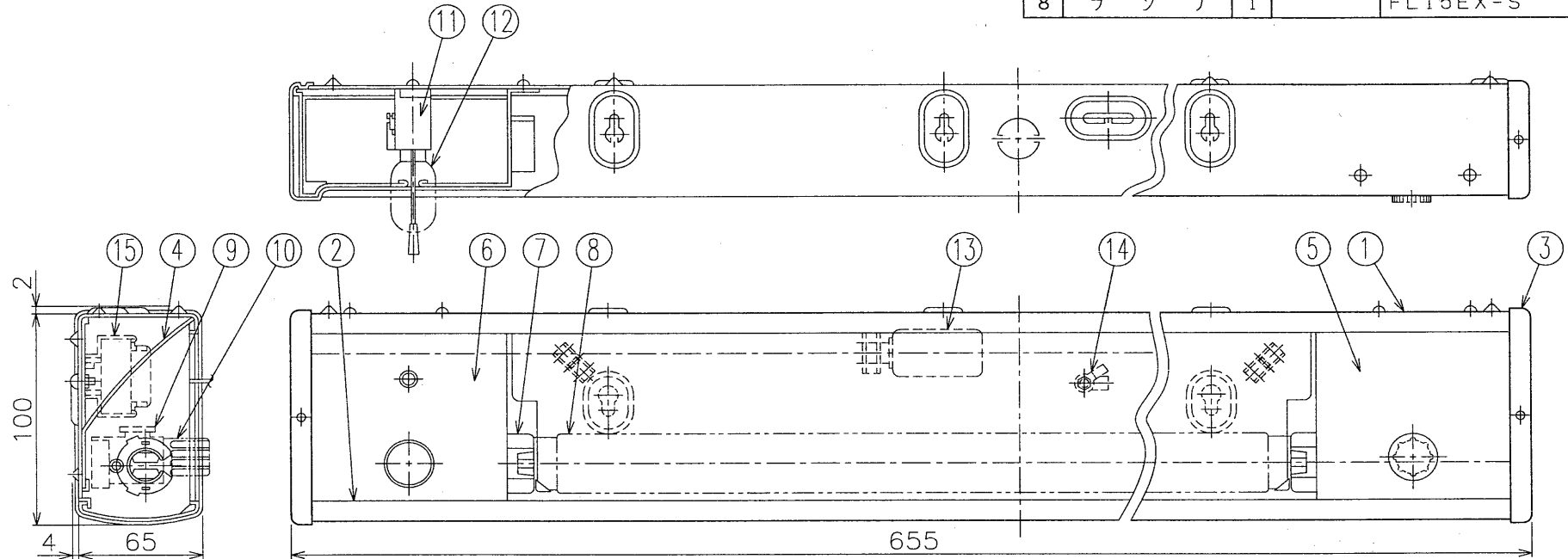
取付寸法図
