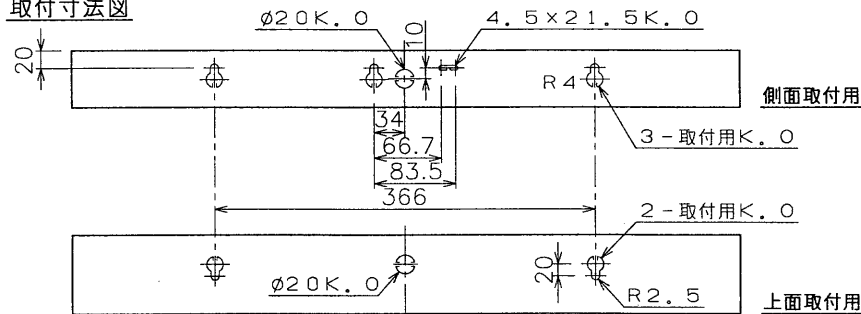
取付寸法図
