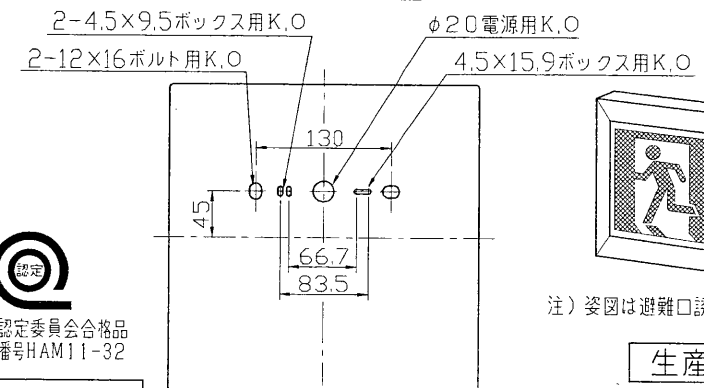
背面取付図
