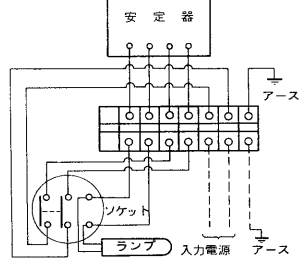
結線図
