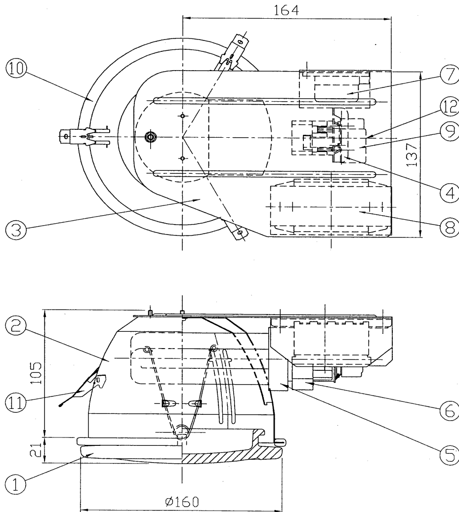
埋込穴寸法 天井取付厚さ：5～24mm
